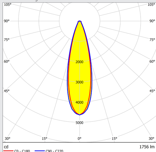
Lichtverteilung mit LED Lextar PC56H19 V1
